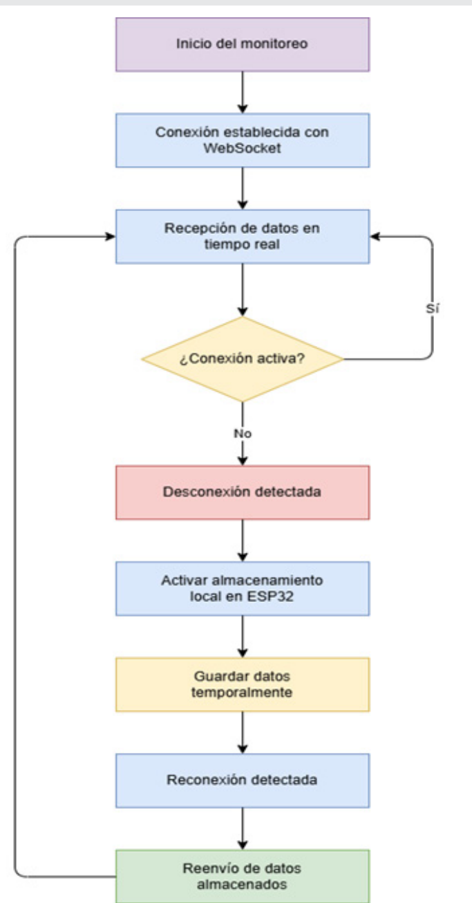
Figura 11: Algoritmo de continuidad de datos durante desconexiones y reconexiones.
